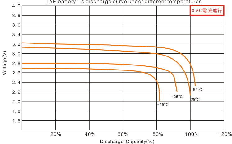
不同環境溫度下LYP類電池的放電特性曲線
